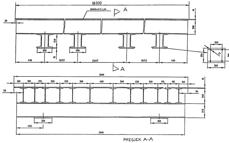
MOSNA KONTRUKCIJA VAGE
