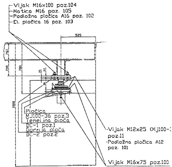
MOSNA KONTRUKCIJA VAGE
